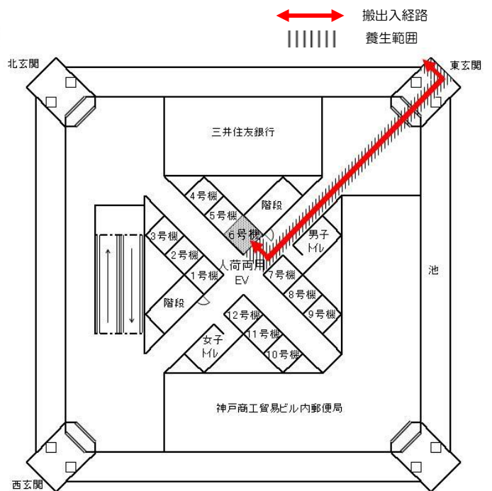
図② 1階 搬出入経路および養生範囲
